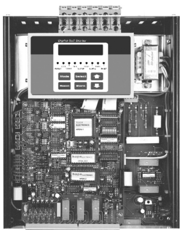
1-3 4-9 10-21 22-24 25-32 Клеммы входов/выходов
